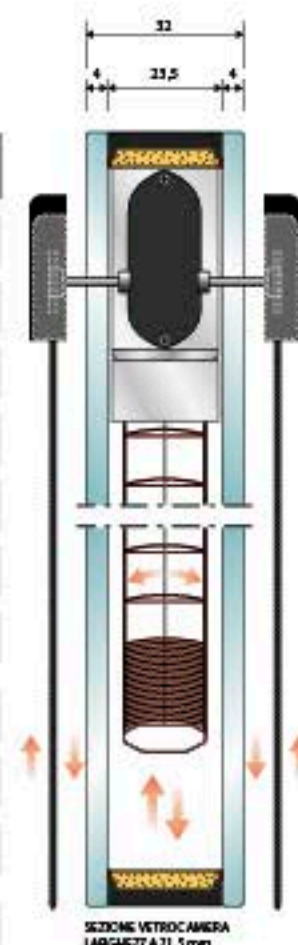
SEZIONE VETROCAMERA LARGHEZZA 23,5 mm
