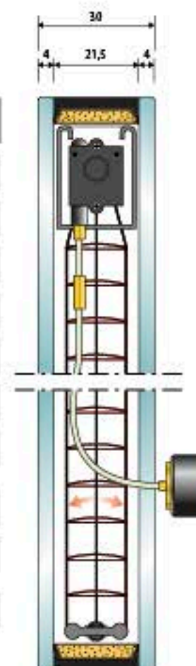
SEZIONE VETROCAMERA LARGHEZZA 21,5 mm
