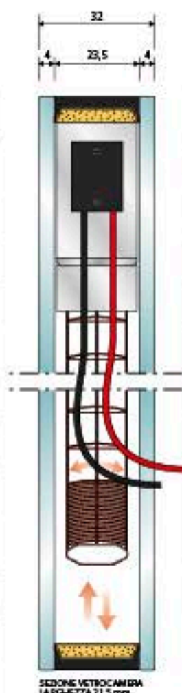
SEZIONE VETROCAMERA LARGHEZZA 23,5 mm
