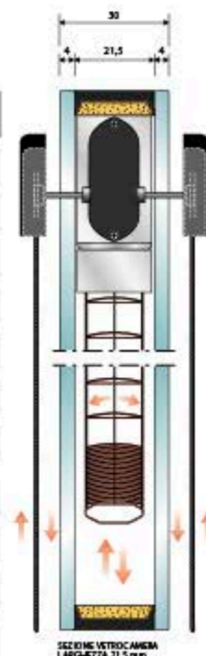
SEZIONE VETROCAMERA LARGHEZZA 21,5 mm
